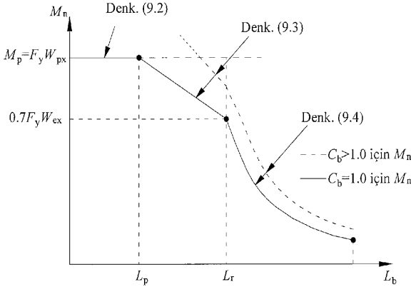
Şekil 9.1 – Basınç başlığının yanal olarak desteklenmeyen uzunluğuna bağlı olarak karakteristlik eğilme momenti dayanımı
